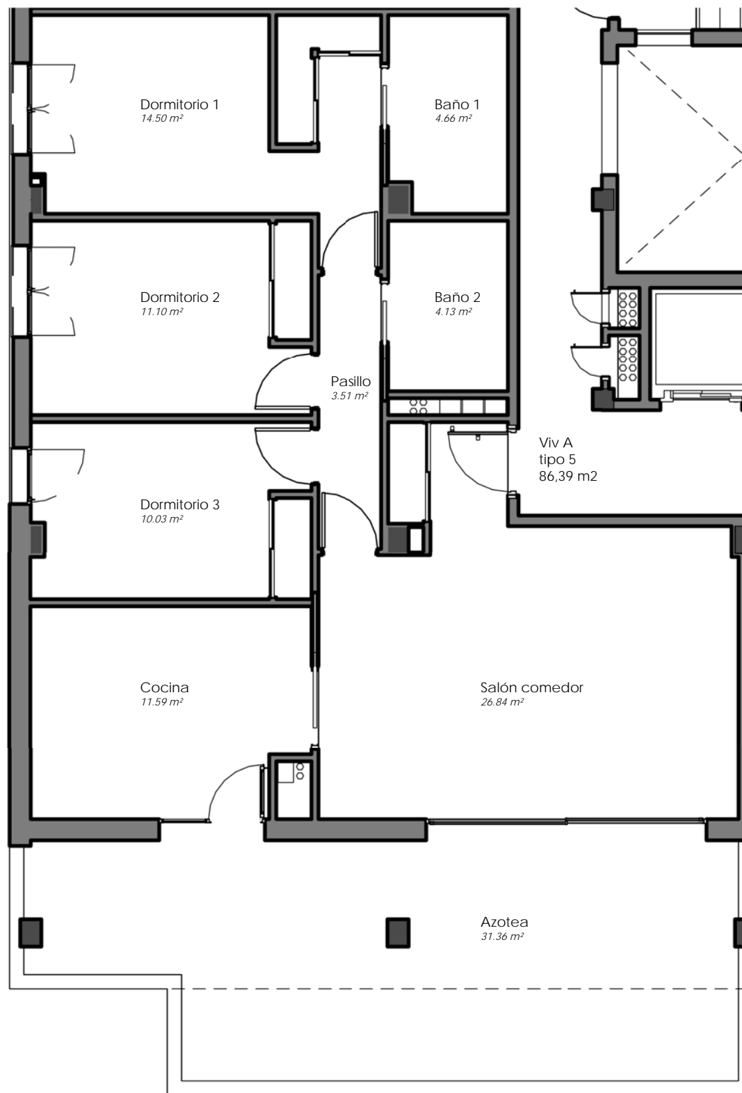
Planta de superficies
