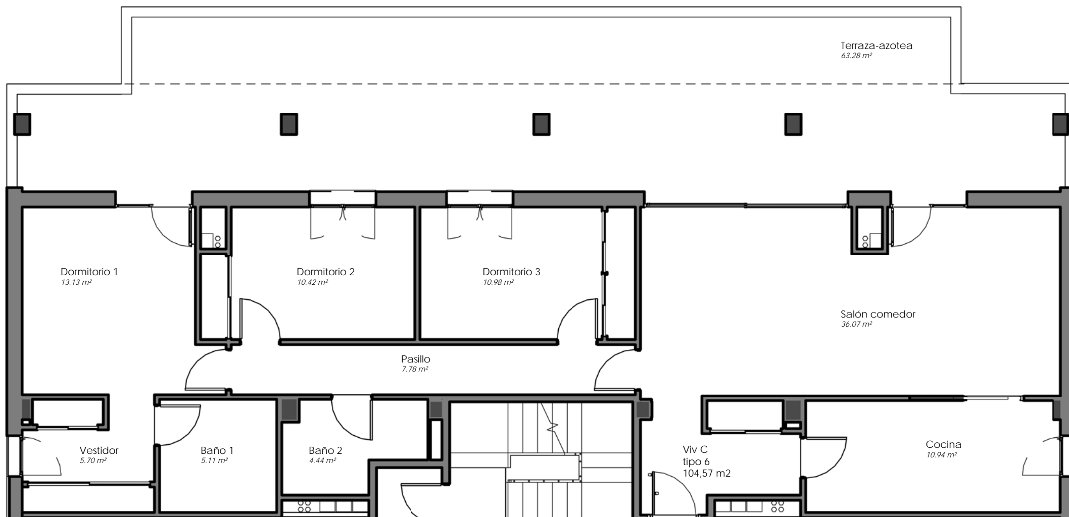
Planta de superficies
